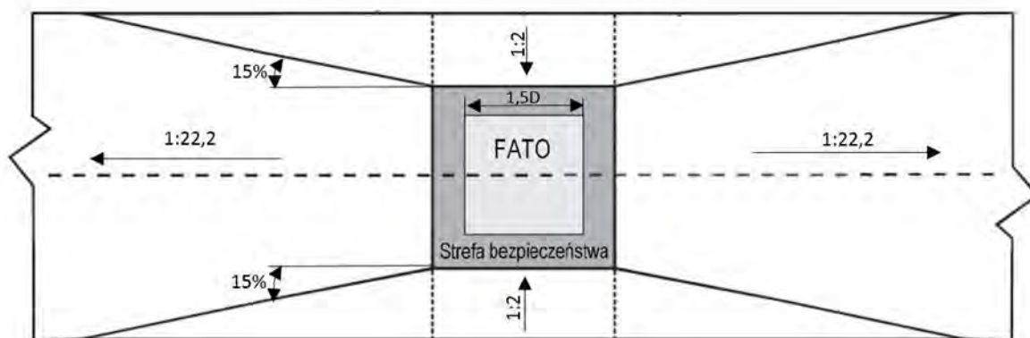
Rzut poziomy
